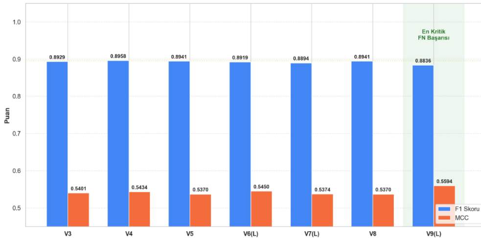
Şekil 2: Versiyon Bazlı Model Karşılaştırması
