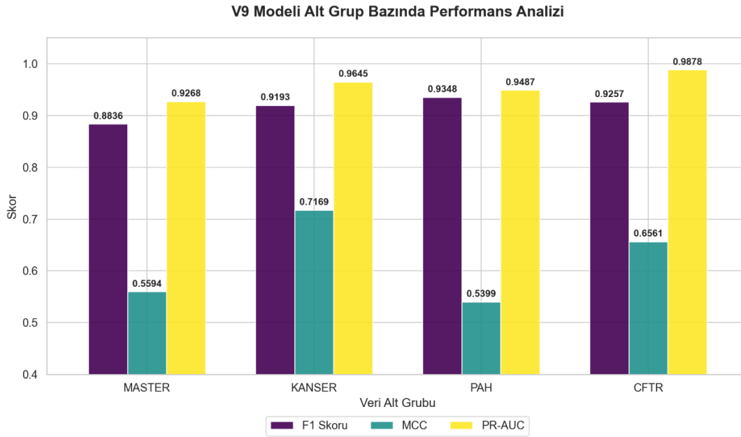
Şekil 3: V9 Modeli — Alt Grup Bazında Performans Analizi (MASTER, KANSER, PAH, CFTR)
