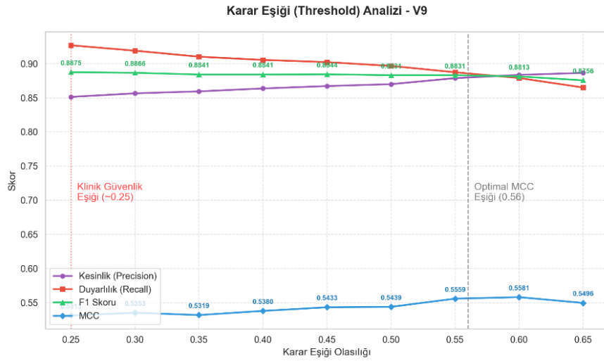
Şekil 5: Karar Eşiği (Threshold) Analizi — V9 Modeli (MASTER)
