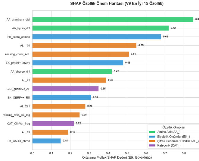
Şekil 1: SHAP Özellik Önlem Analizi (V9) – En Önemli 15 Özellik
